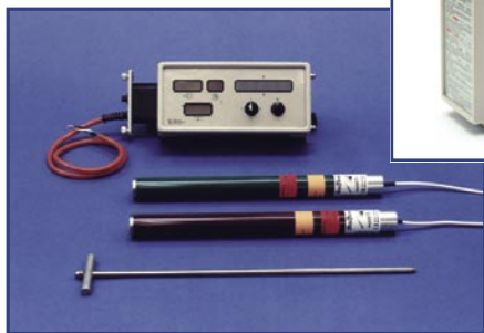
Приемник Mark III (наверху) и кабельная система (слева) сверху вниз: выносной дисплей для работы с кабельной системой и источник питания, стандартный и высокочувствительный к углу наклона кабельный излучатель, инструмент DCI для установки/извлечения.
