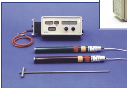
Mark III Empfänger (oben) und Kabelsystem (links), von oben nach unten, Fernanzeige inkl. Kabelfunktion mit Stromversorgung, Standard-Transmitter und 0.1% Transmitter. Ein- / Ausbau Werkzeug
