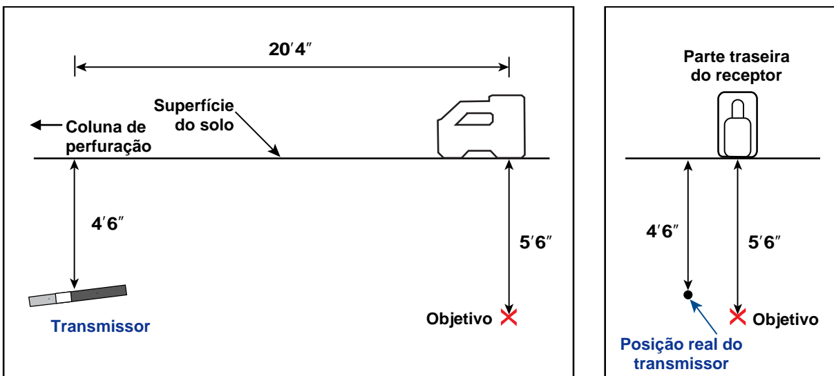
Vista lateral e vista traseira mostrando o posicionamento do receptor, transmissor e objetivo
