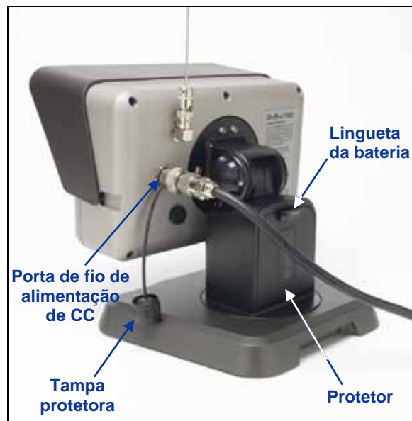
O cabo de alimentação de CC e o protetor instalados no remoto FSD
