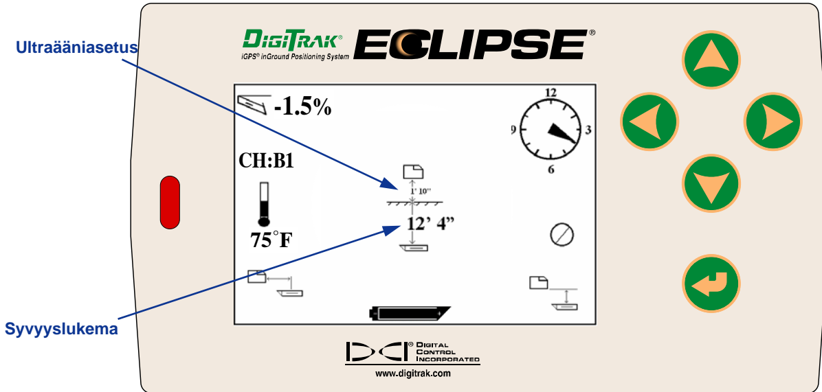
Syvyyss näyttö etänäytössä (vastaanotin LL-pisteen yläpuolella)
