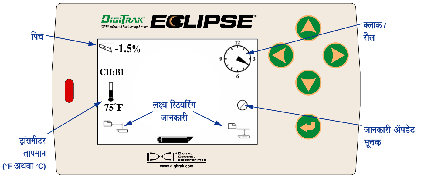
रिमोट डिसप्ले स्क्रीन (जबकि रिसेवर FLP, RLP, अथवा LL के ऊपर न हो)
