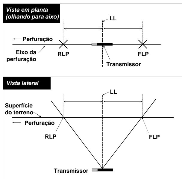
Vista Emplanta e Lateral do FLP, RLP, e LL Quando o Transmissor Está Estável Nivelado com o Solo
