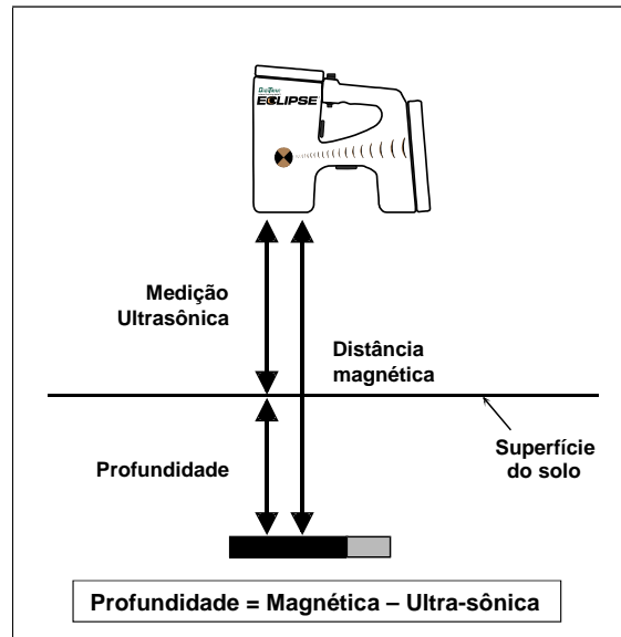
Uso da Medição Ultrasônica para Determinar a Profundidade Real
