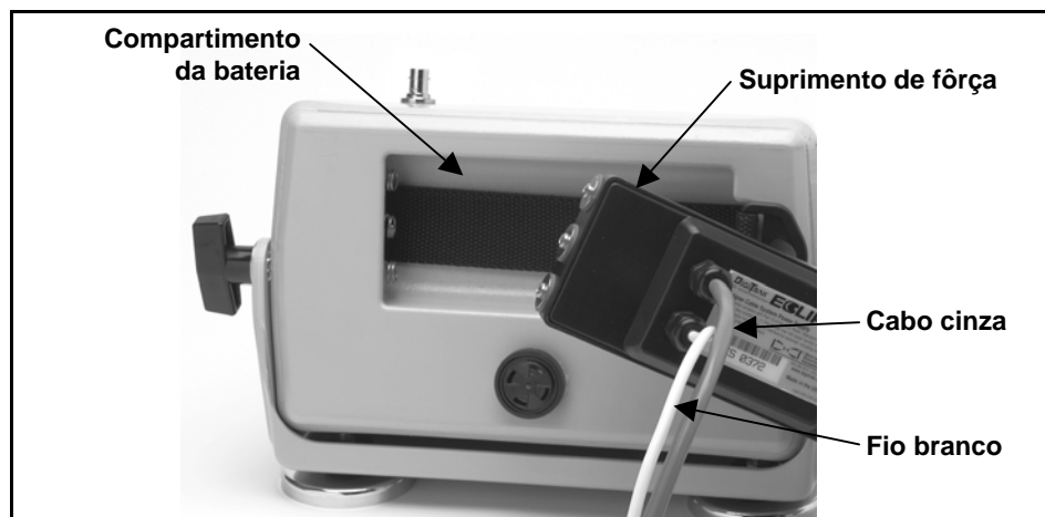
Fornecimento de Suprimento de Fôrça ao Contrôle Remoto
