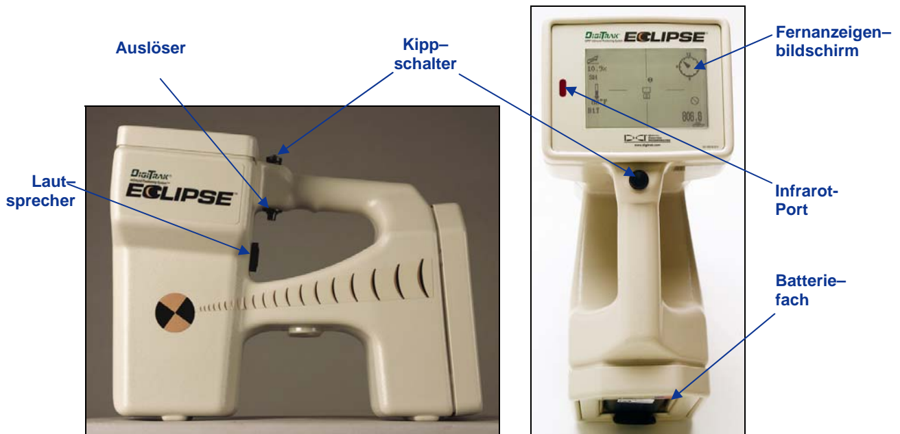
Eclipse Empfänger: Seitenansicht (links) und Ansicht von oben (rechts)
