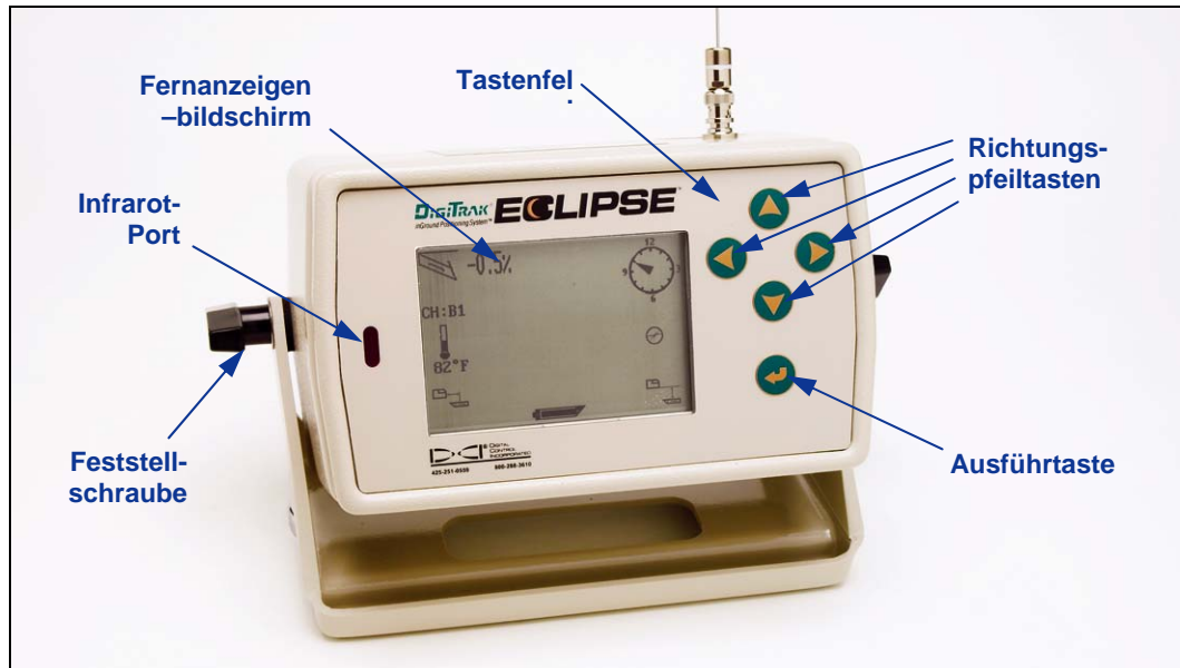
Eclipse Fernanzeige
