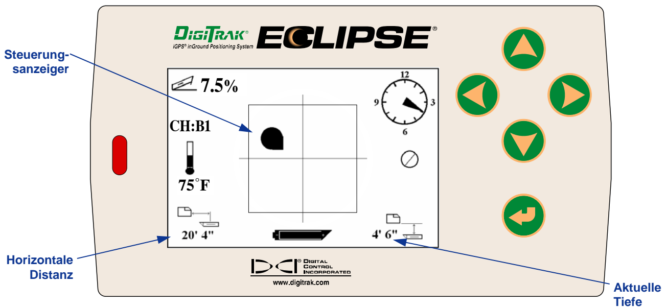
Target Steering Anzeigefenster an der Fernanzeige
