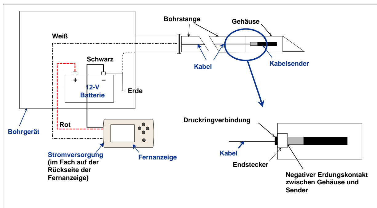
Anschluss der Kabelsystemkomponente
