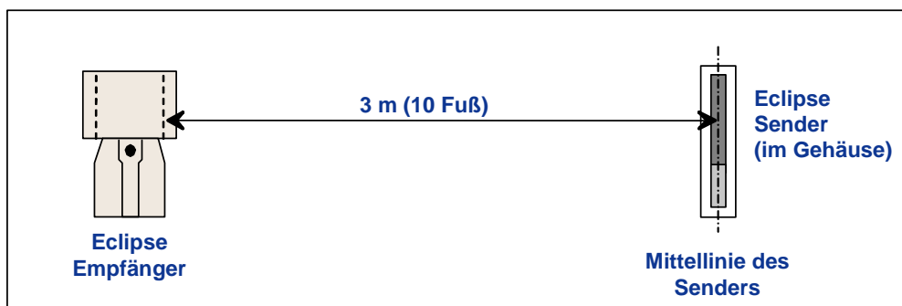
3 m (10 Fuß) Abstand für die 1-Punkt-Kalibrierung
