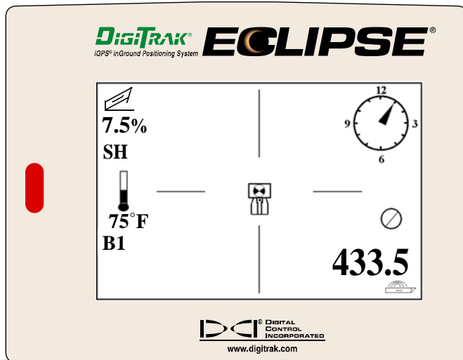
Eclipse Ortungsanzeige, während sich das Ziel am FLP in der Box befindet
