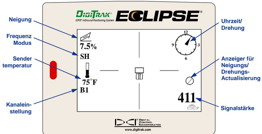
Bildschirm des Ortungsmodus
