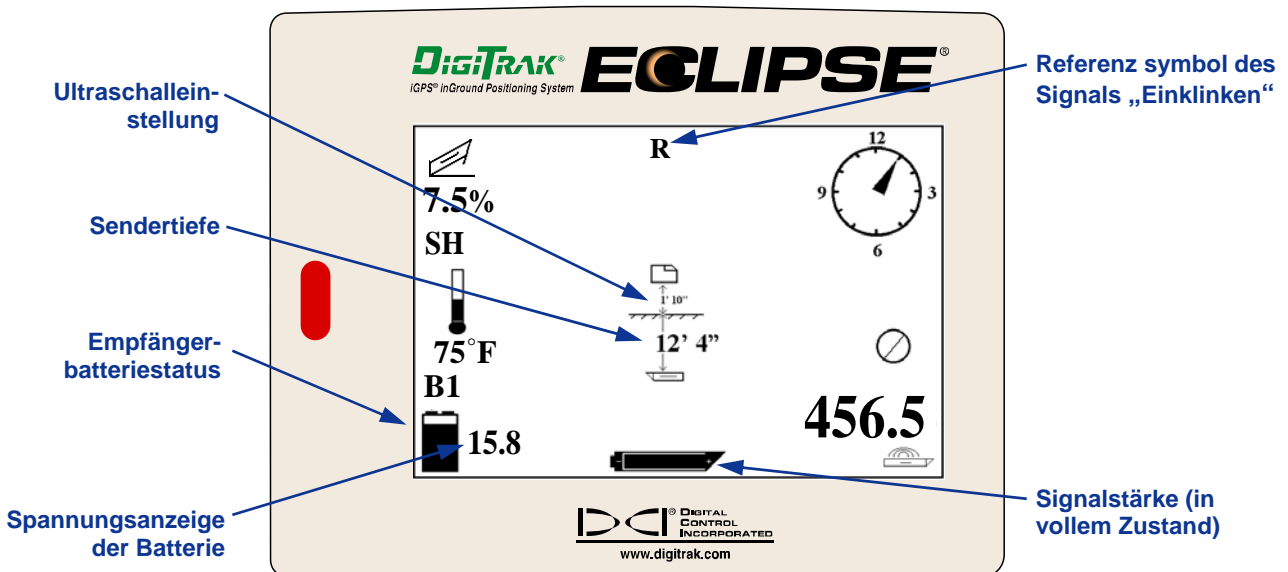
Bildschirm zur Tiefendarstellung
