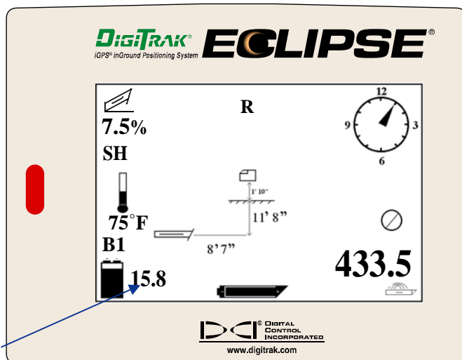
Eclipse Anzeige zur vorgesehenen Tiefe
