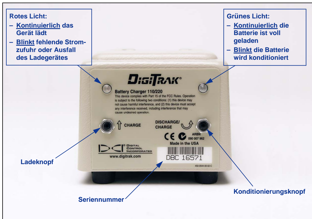
Instrumententafel des Batterieladegerätes
